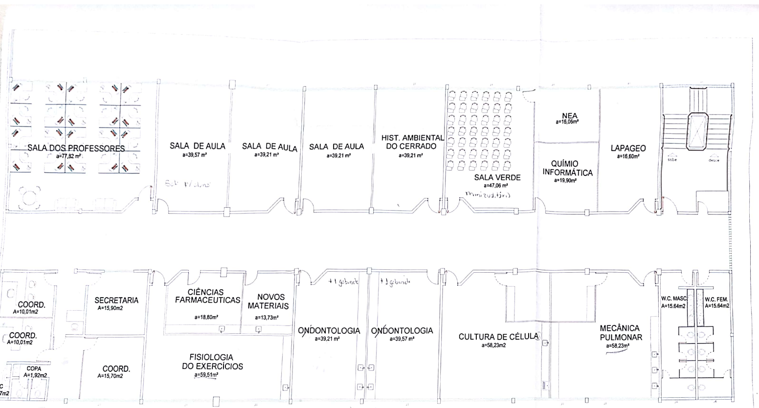
PLANTA BAIXA, 4º PAV., BLOCO "B" - Area=1.226,60m 2 (PROPOSTA PÓS GRADUAÇÃO)
